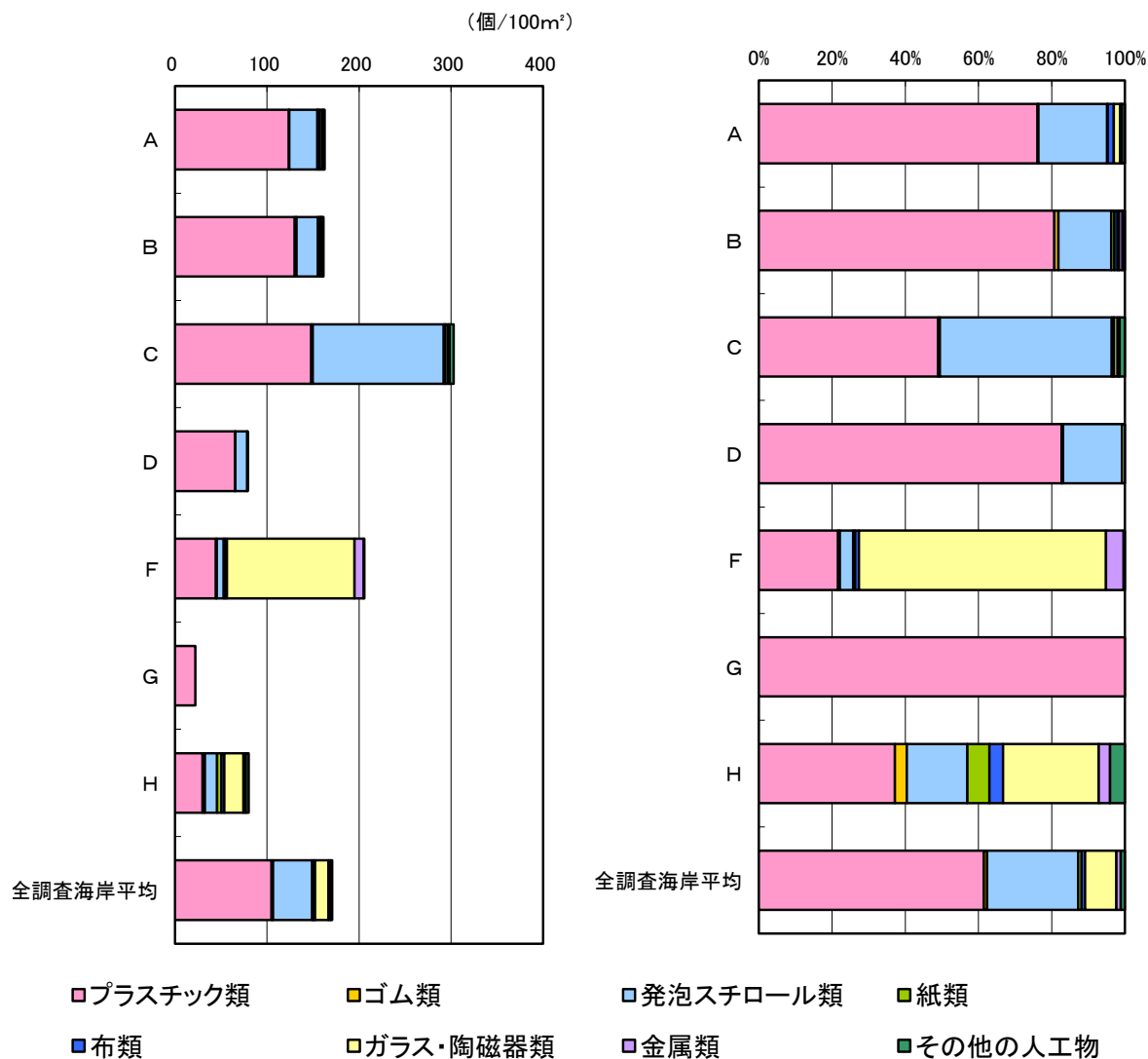
図2. 4-3 エリア別単位面積あたりの漂着物個数(個/100m 2 )と割合(%)
