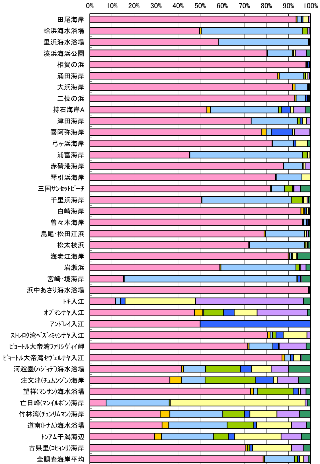
図2. 2-7 2018年度 海岸別単位面積あたりの漂着物個数の組成比率(%)
