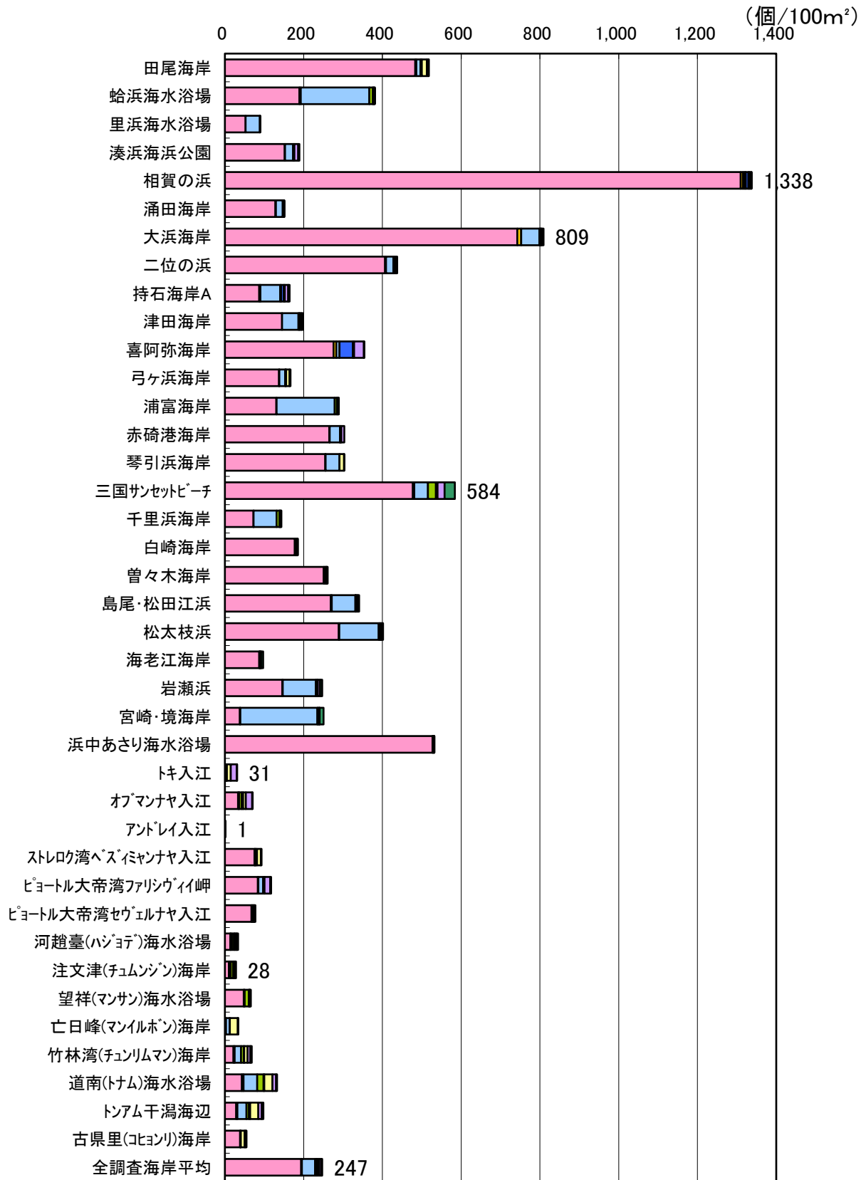
図2. 2-5 2018年度 海岸別単位面積あたりの漂着物個数(個/100m 2 )
