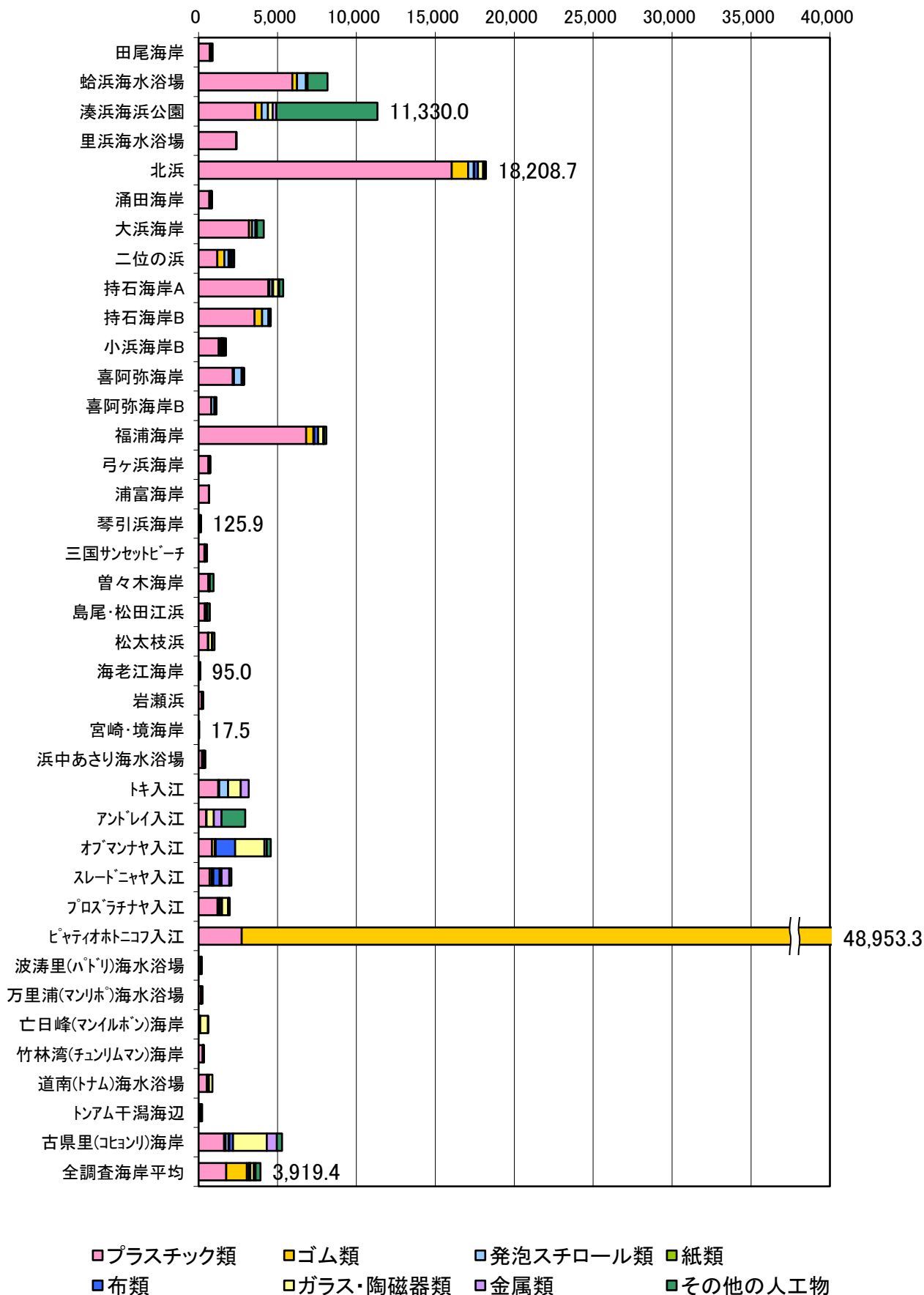
図2. 2-1 海岸別単位面積あたりの漂着物重量(g/100m 2 )
