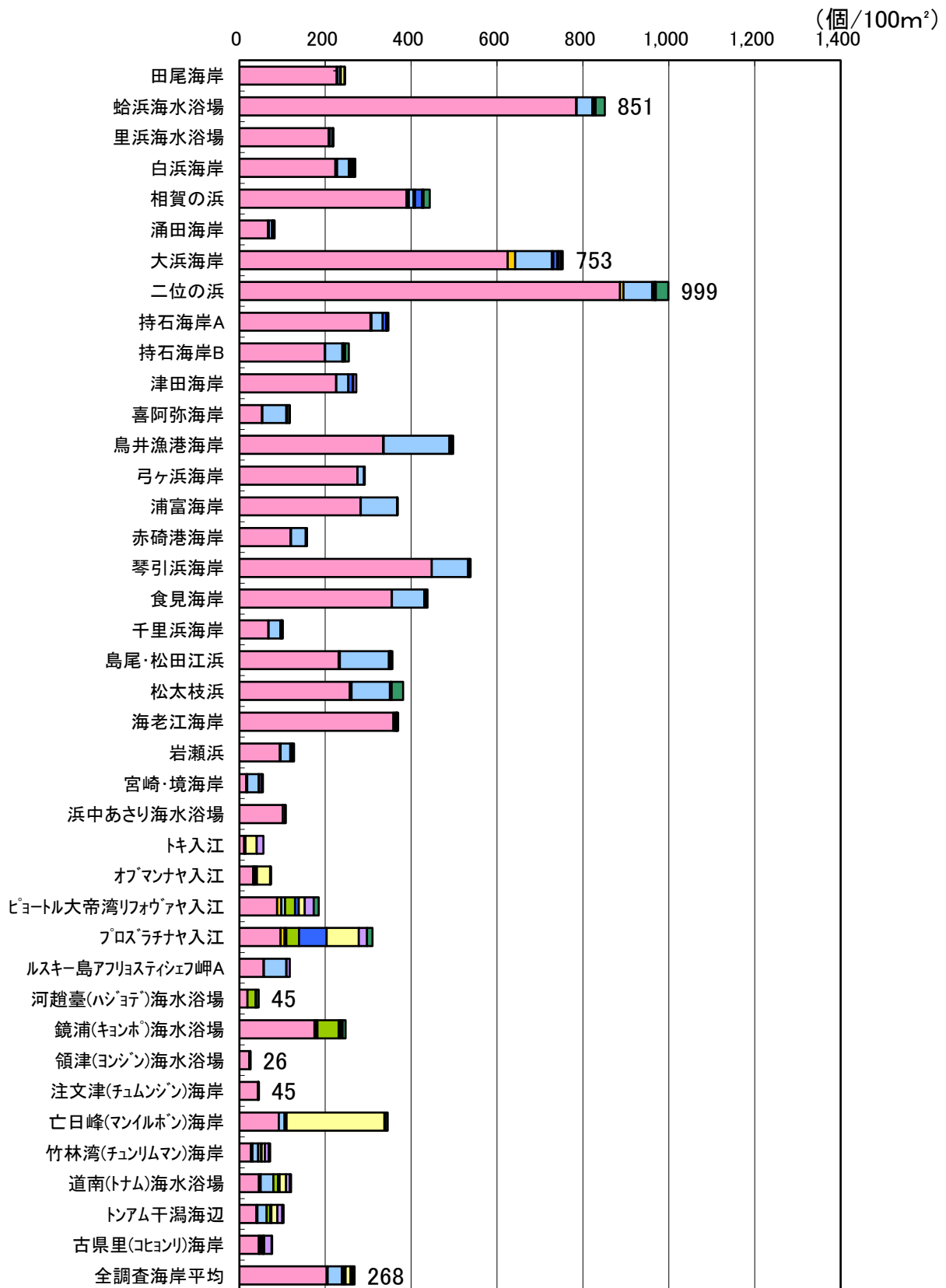
図2. 2-5 2019年度 海岸別単位面積あたりの漂着物個数(個/100m 2 )
