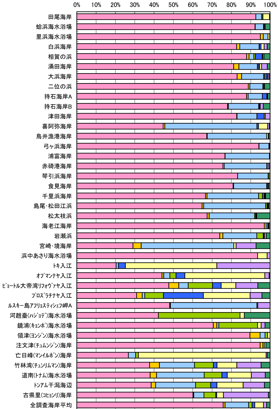
図2. 2-7 2019年度 海岸別単位面積あたりの漂着物個数の組成比率(%)
